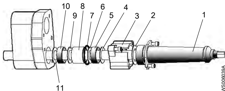
Рис. 22: Блоки привода 605-776
