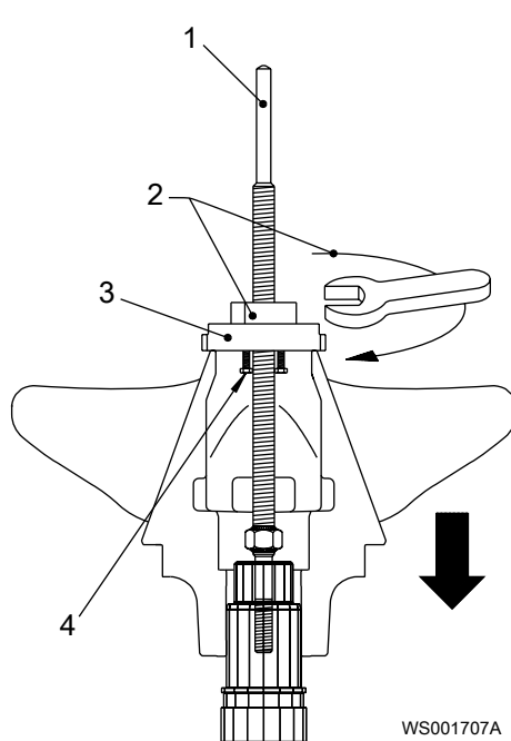
Рис. 49: P7061
