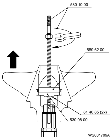
Рис. 48: P7061
