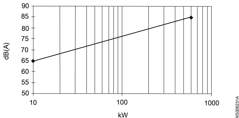
Рис. 37: Звуковое давление
