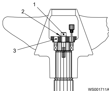
Рис. 52: P7081
