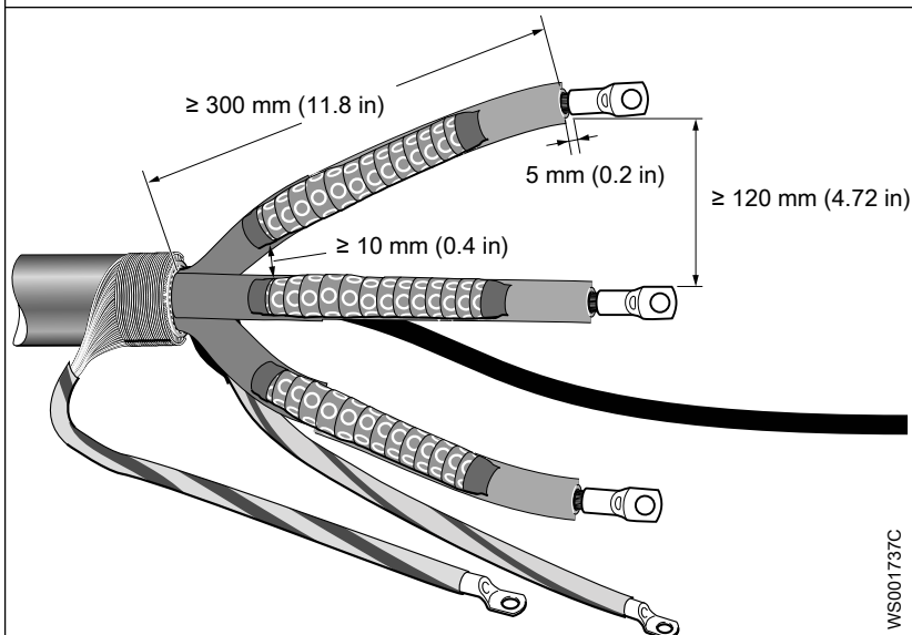
Рис. 32: Рекомендуемые расстояния
