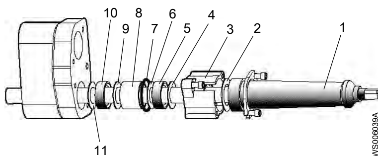
Рис. 18: Блоки привода 605-776
