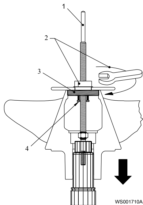
Рис. 50: P7081
