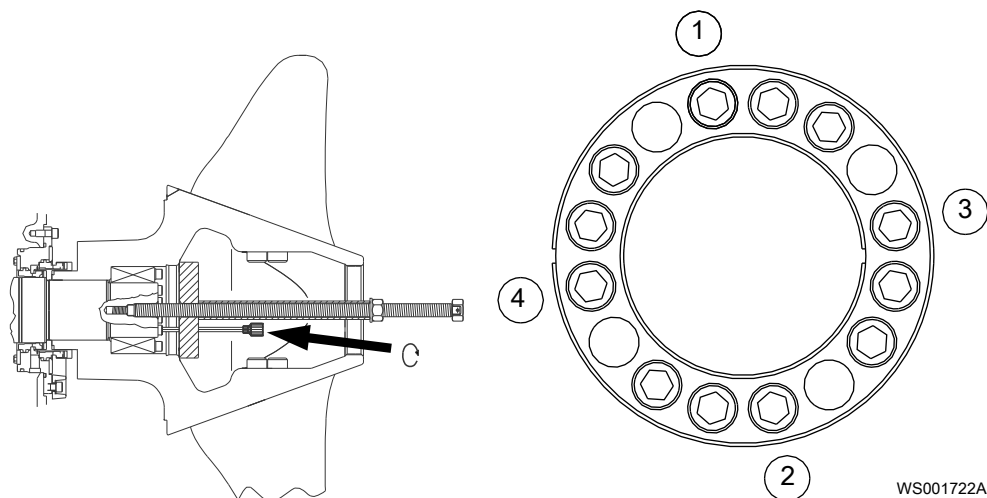
Рис. 58: P7121/965-998
